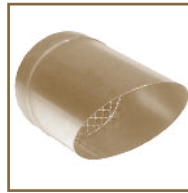
BUSE BIÈAUTÉE GRILLAGÉE réf. BBG Fonction : protection pare-pluie et anti-volatile du rejet horizontal (HH) des caissons placés en extérieur. Diamètre des piquages : 315, 450 et 500 mm.
